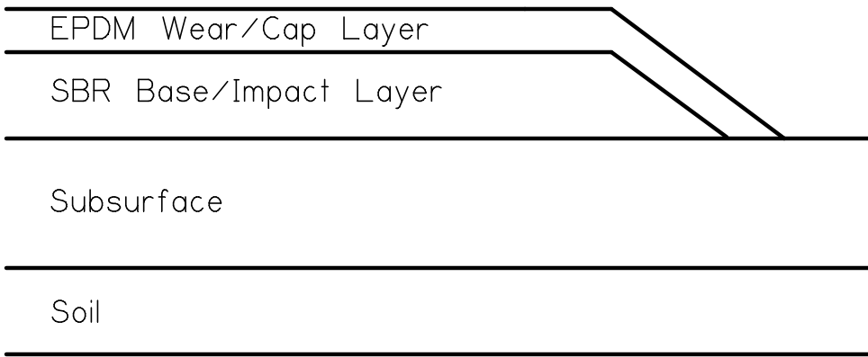
Beveled Edge
